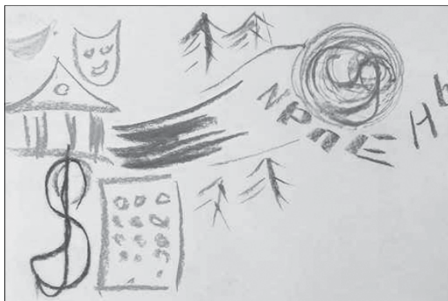
Рис. 2. Ментальна мапа
