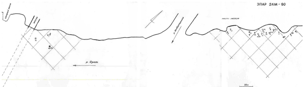
Рис. 1. Рельєф дна та лінія правого берега Орилі в районі впадіння Нехворощанки з позначками місць археологічних знахідок
